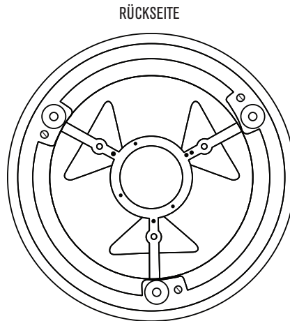
V Hauptspiegel in der Spiegelzelle
